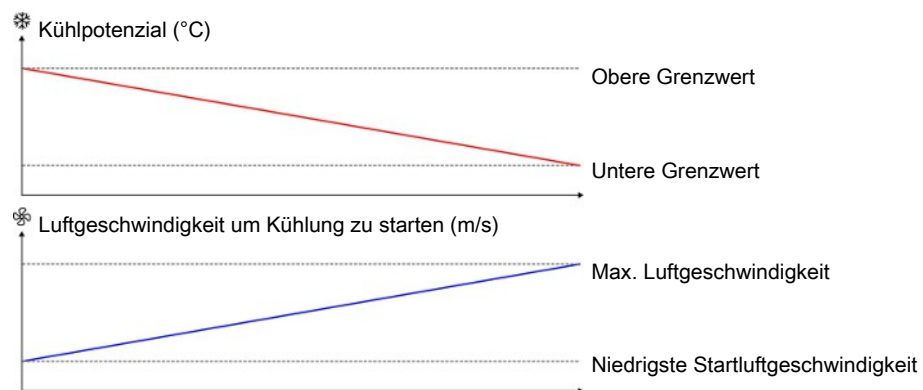
Abb. 31: In Bereichen mit geringer Außenluftfeuchte und großem Kühlpotenzial kann die Kühlung mit einer niedrigeren Luftgeschwindigkeit beginnen. In Bereichen mit geringem Kühlpotenzial beginnt die Kühlung dagegen so spät wie möglich, d. h. bei maximaler Luftgeschwindigkeit.
