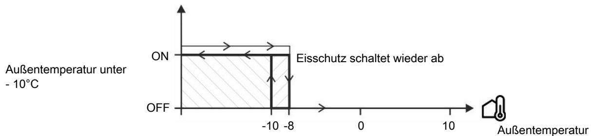
Abb. 13: Aktivierung von Eisschutz
