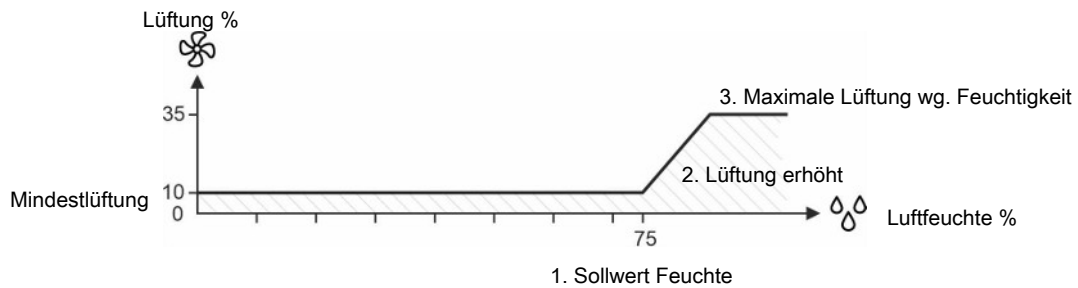
Abb. 11: Feuchtelüftung: 1. Die Luftfeuchtigkeit überschreitet den Feuchte-Sollwert. 2. Lüftung wird vom Stallcomputer verstärkt. 3. Steigerung bis zur maximalen Feuchtelüftung (35%).
