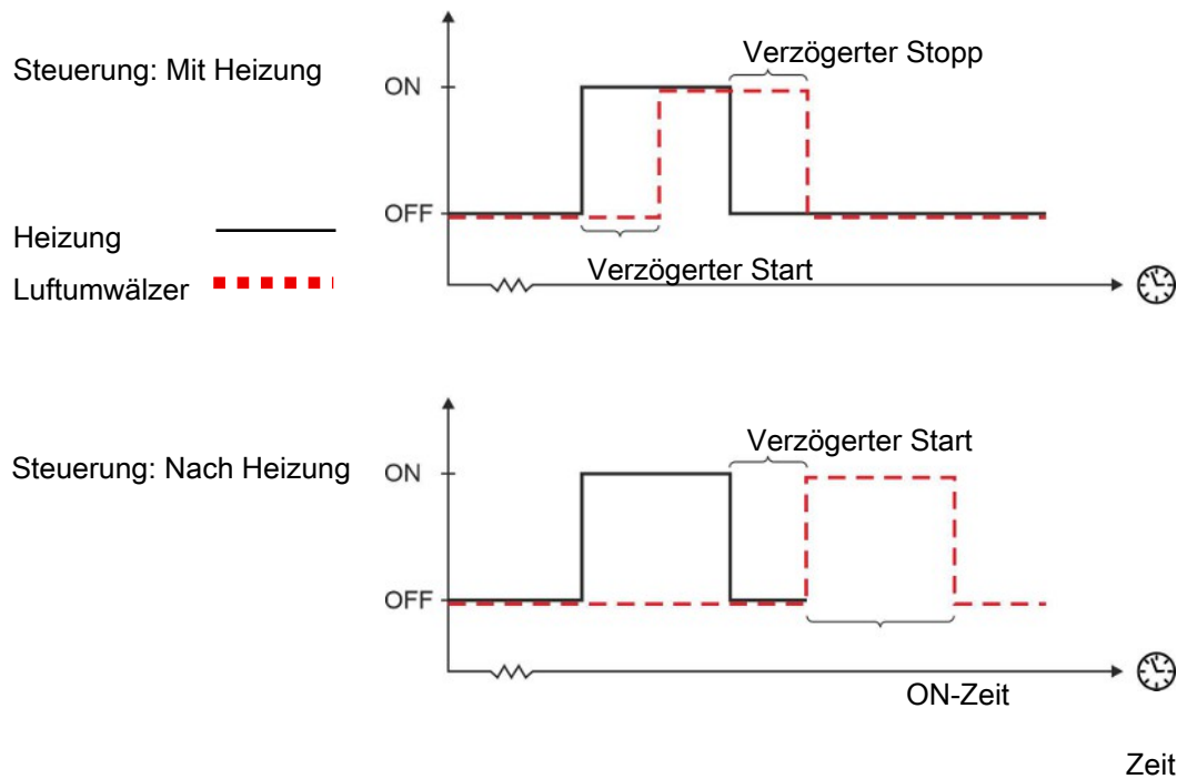
Abb. 23: Steuerung durch Heizquelle
