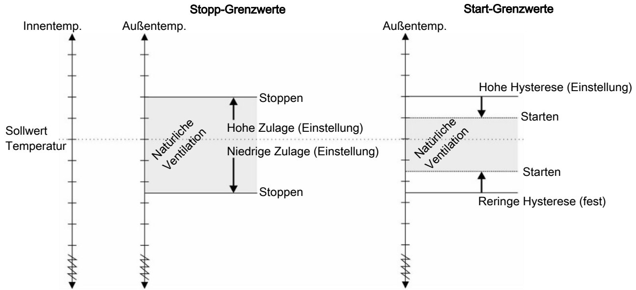
Abb. 20: Start und Stopp in Abhängigkeit von der Außentemperatur. Die Temperaturgrenzen werden als Abweichung vom Temperatursollwert festgelegt.
