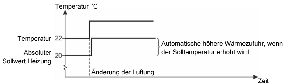
Abb. 34: Wärmezufuhr
