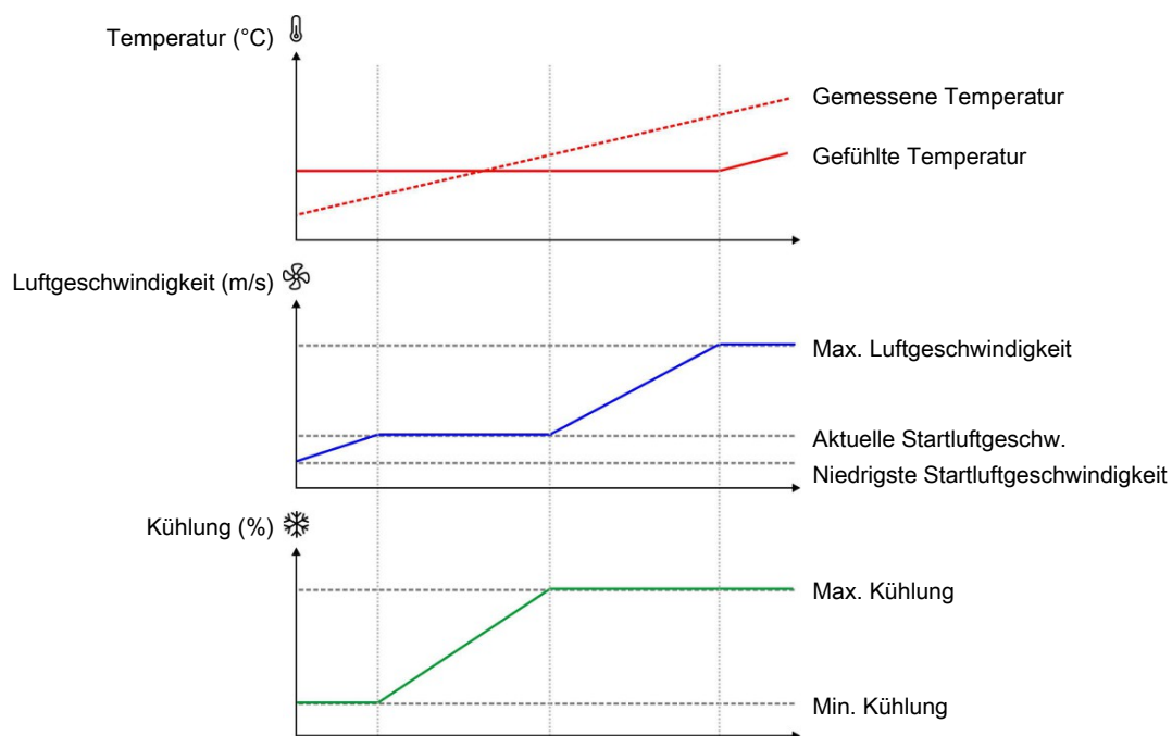
Abb. 32: Die Kühlung startet bereits bei niedriger Luftgeschwindigkeit, um die erforderliche Innentemperatur zu halten. Wenn die Kühlung die Temperatur nicht halten kann, wird die Luftgeschwindigkeit wieder erhöht.
