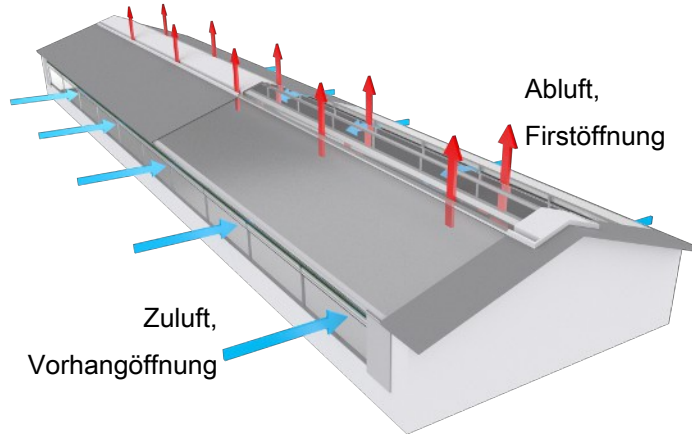
Abb. 17: Beispiel: auf einem Stall nur mit natürlicher Ventilation mit Vorhangöffnungen an den Seiten des Stalls und Firstöffnung auf dem Dach
