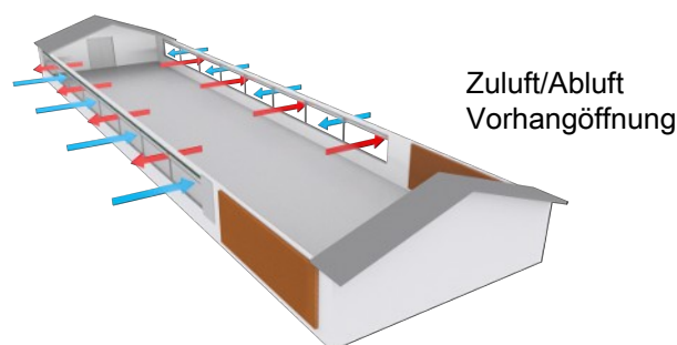
Abb. 18: Stallbeispiel mit Natürlicher Ventilation in Kombination mit Tunnellüftung, Natürliche Ventilation.
