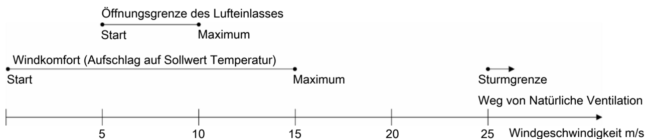
Abb. 21: Natürliche Ventilation bei zunehmender Windgeschwindigkeit
