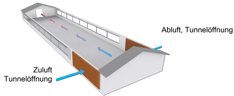
Abb. 19: Beispiel für einen natürlich belüfteten Stall in Kombination mit Tunnel-Lüftung.
