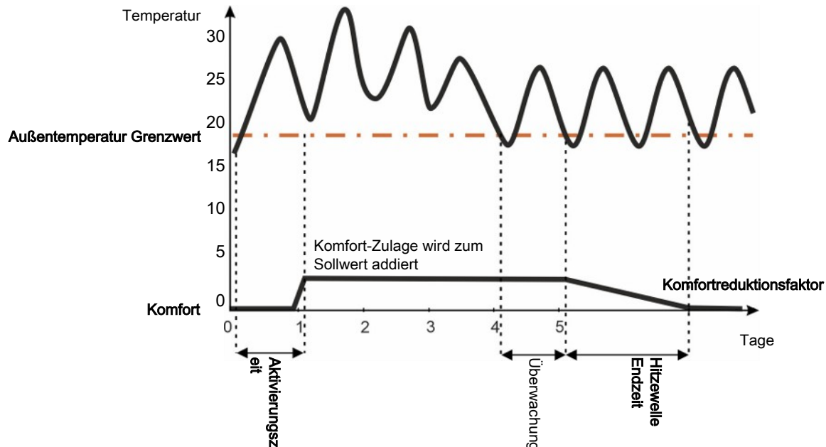
Abb. 5: Hitzewelle Komfort
