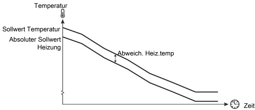
Abb. 33: Abweich. Heiz.temp
