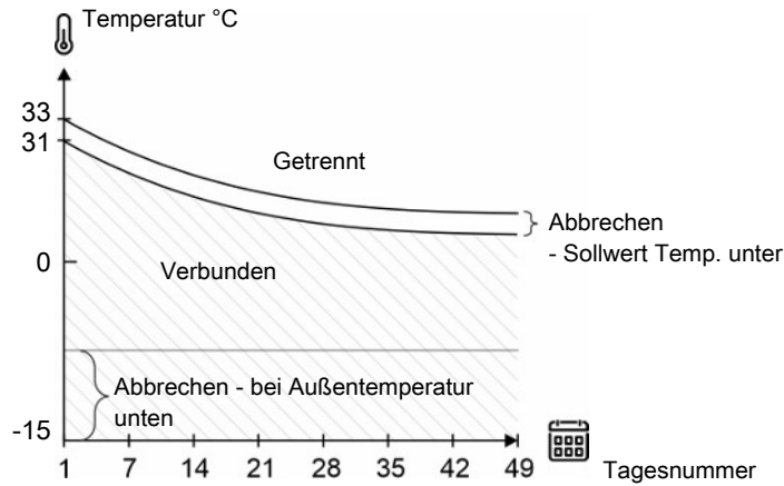
Abb. 15: Wärmetauscher – niedrige und hohe Außentemperaturgrenze
