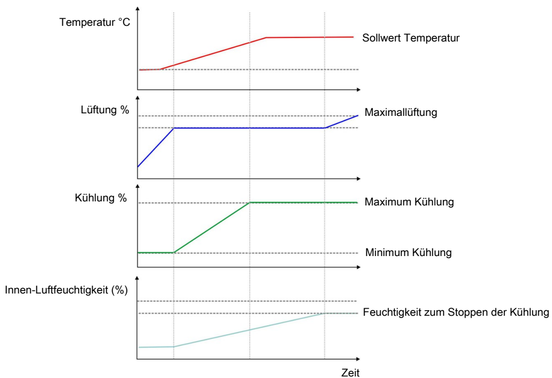
Abb. 25: Um die geforderte Innentemperatur zu halten, beginnt die Kühlung, bevor das Lüftungsniveau die Maximallüftung erreicht hat. Wenn die Kühlung die Temperatur nicht halten kann, wird die Luftgeschwindigkeit wieder erhöht.
