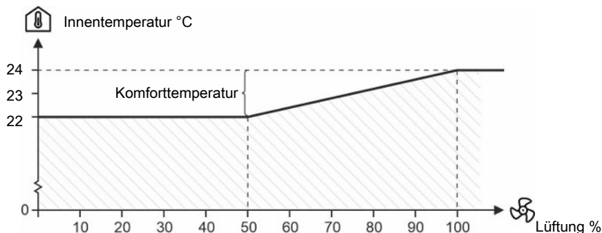
Abb. 7: Komforttemperatur bei kontinuierlichem Betrieb
